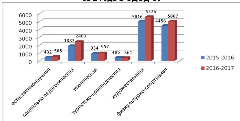
Сравнительная диаграмма распределения направленностей за 2 года в ОДОД ОУ
